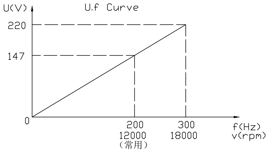
频压曲线
