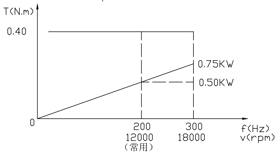
扭矩/功率曲线
